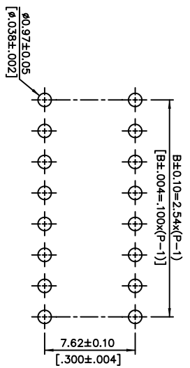
P.C.B. LAYOUT
